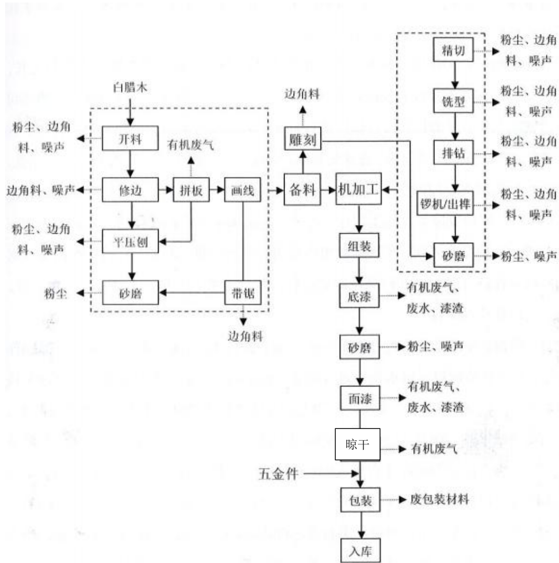
图 3-1 生产工艺流程及产污环节图
